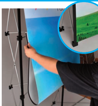
Nun mit beiden Händen die Druckbahn straff halten und gleichmäßig stückweise auf die Metallbahn fallen lassen. Den Druck möglichst mittig auf der Metallschiene ausrichten.
